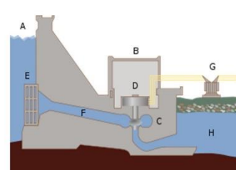
Az erőmű felépítése
